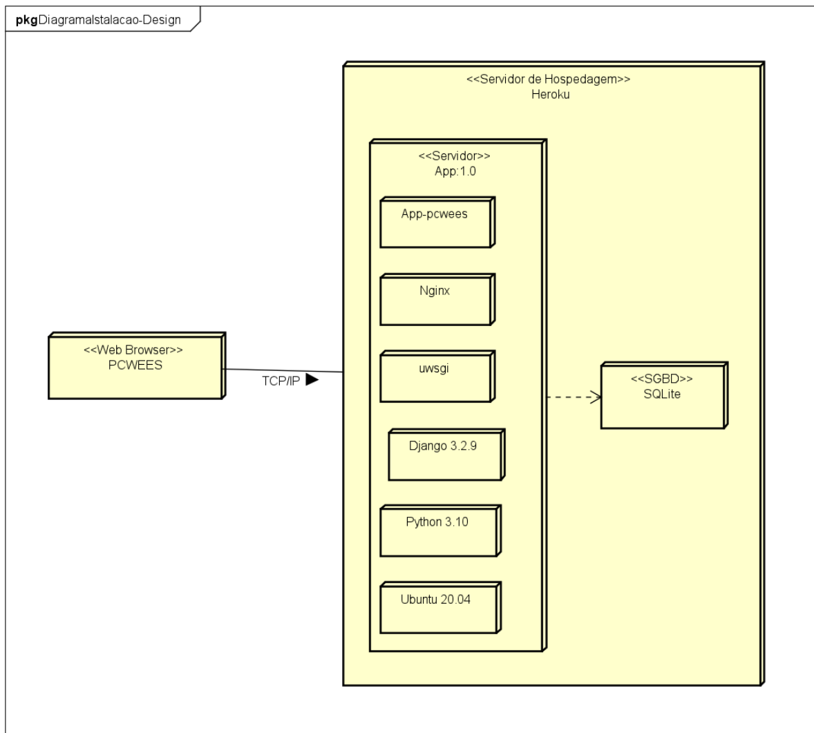
Figura 55 - Modelo de instalação do PCWEES
